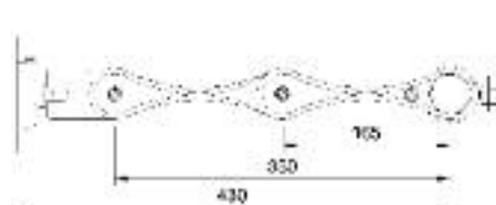
Art.nr. 6FSA8503000 Sidewinder Mini/Maxi LCD arm QR , max./min. uitslag 357/99mm.
