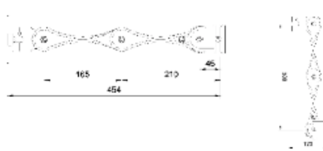
Art.nr. 6FSA8741.675 Sidewinder Slatwall Maxi/Maxi LCD arm, max./min. uitslag 454/123mm.
