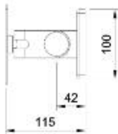
Art.nr. 6FSA6143.675 CopperHead Slatwall QR Mini LCD arm, max./min. uitslag 115/42mm.
