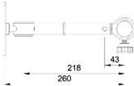
Art.nr. 6FSA6203000 Viper Midi QR LCD arm, max./min. uitslag 260/119mm
