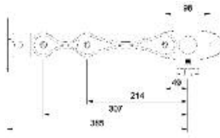
Art.nr. 6FSA8561005 Sidewinder Dubbele Mini/Maxi LCD arm, max./min. uitslag 307/214mm.*
