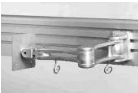
Art.nr. 6FSA8741.675 Sidewinder Slatwall Maxi/Maxi LCD arm, max./min. uitslag 454/123mm.
