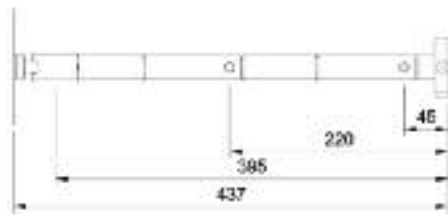
Art.nr. 6FSA6243675 Viper Slatwall QR Midi LCD arm, max./min. uitslag 262/114mm.
