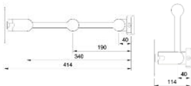
Art.nr. 6FSA6743.675 CopperHead Slatwall QR Maxi LCD arm, max./min. uitslag 414/114mm
