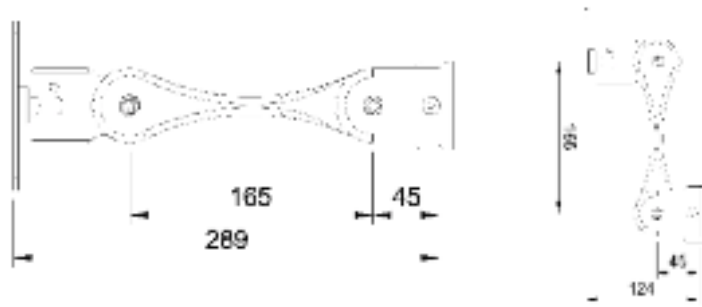
Art.nr. 6FSA8341.675 Sidewinder Slatwall Midi LCD arm, max./min. uitslag 289//124mm
