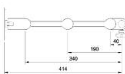
Art.nr. 6FSA6301000 CopperHead Midi LCD arm, max./min. uitslag 264/74mm.
