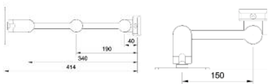
Art.nr. 6FSA6343.675 CopperHead Slatwall QR Midi LCD arm, max./min. uitslag 269/119mm.
