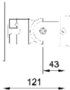
Art.nr. 6FSA8143.675 Sidewinder QR Slatwall Mini LCD arm, max./min. uitslag 121/43mm.
