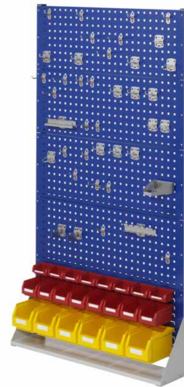
Type-5: hoogte 1790mm. 4 geperf.-/ 1 sleuvenpaneel.
