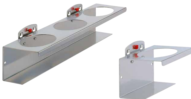
Houder voor spuitbussen etc., met diameter 70mm., L-100/300mm. 1 bus Art.nr. 4042.00.1101 3 bussen Art.nr. 4042.00.1201
