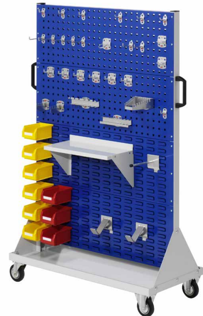
RasterMobil type 4 Grote-4: H: 1580mm. Paneeluitvoering: Gaten Sleuven Gentiaanblauw 8 --- 7022.00.3416 6 2 7022.00.3716 4 4 7022.00.3916 2 6 7022.00.4116
