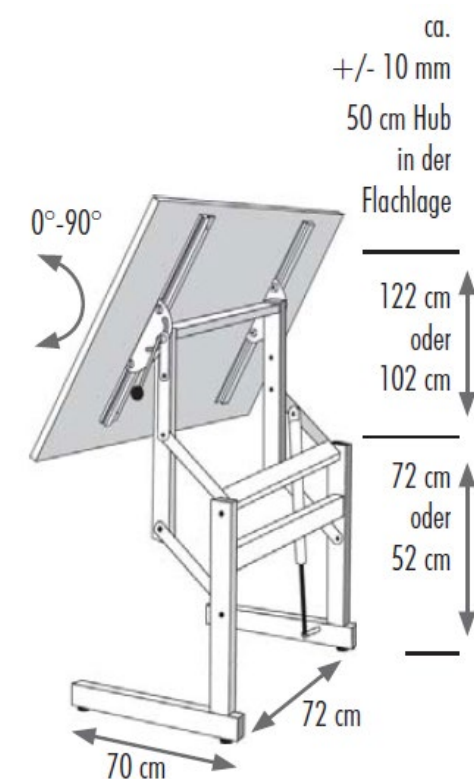
Ergo P1 met T-voet frame 70cm. afhankelijk bladdiepte.
