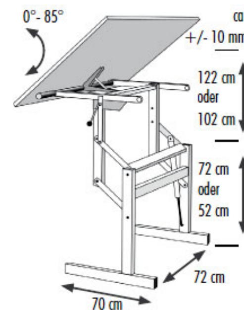
Ergo P1R met C-voet frame 70cm. afhankelijk van blad-diepte geschikt voor rolstoel.
